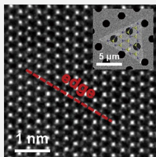
HADF-STEM 图像
